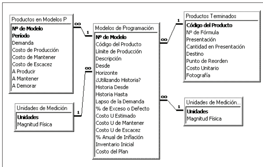
Figura 2. Composición y relaciones de la base de datos
