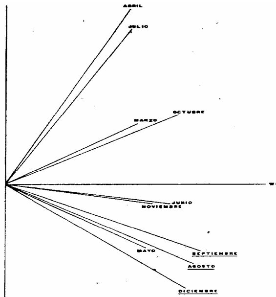
GRAFICO 1. REPRESENTACION GRAFICA DE LA INTERESTRUCTURA (RELACION GRAFICA ENTRE LAS TABLAS-MESSES CON RESPECTO AL COMPROMISO WD).
